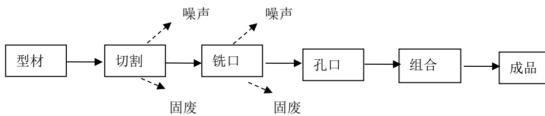
图 2-4 高级门窗生产工艺流程及产污环节图
