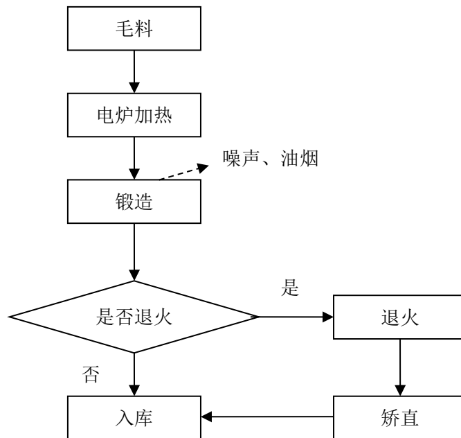
图 2-4 运营期产污环节图
