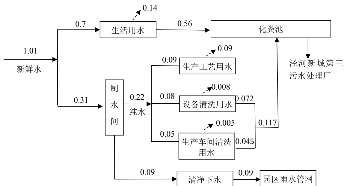
图 2 项目水平衡图 单位: \text{m}^3/\text{d}
