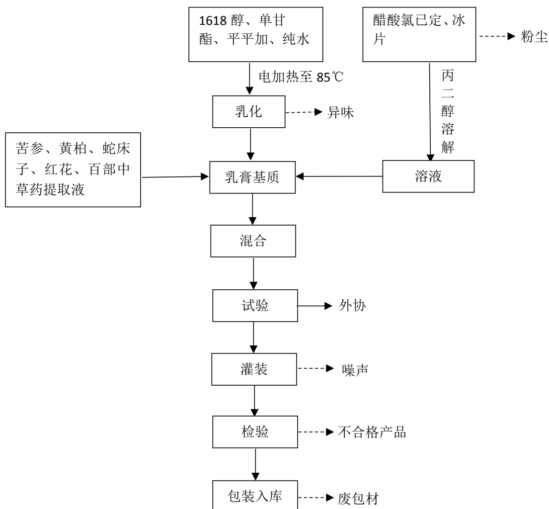
图 3 抑菌乳膏生产工艺流程及产污环节图
