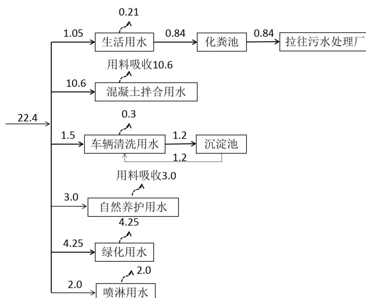
图 1 建设项目水平衡图 (m³/d)
