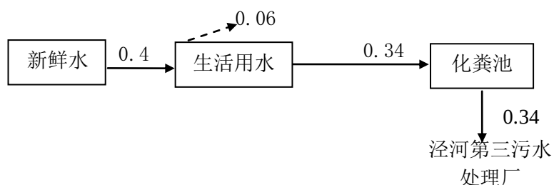
图3 项目水量平衡图 (单位: \text{m}^3/\text{d} )
