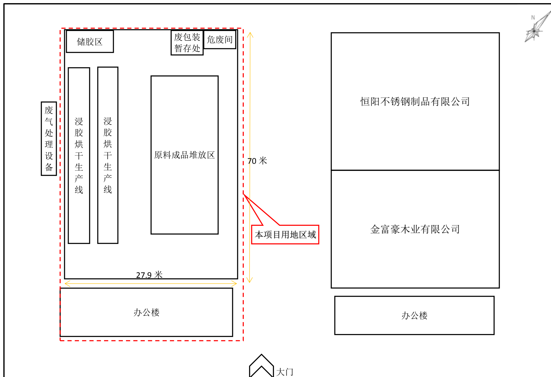
附图五 项目平面布置图
