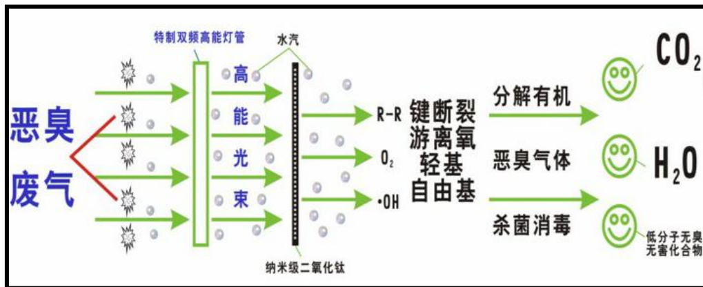
图 3 光氧设备工作工作原理图
