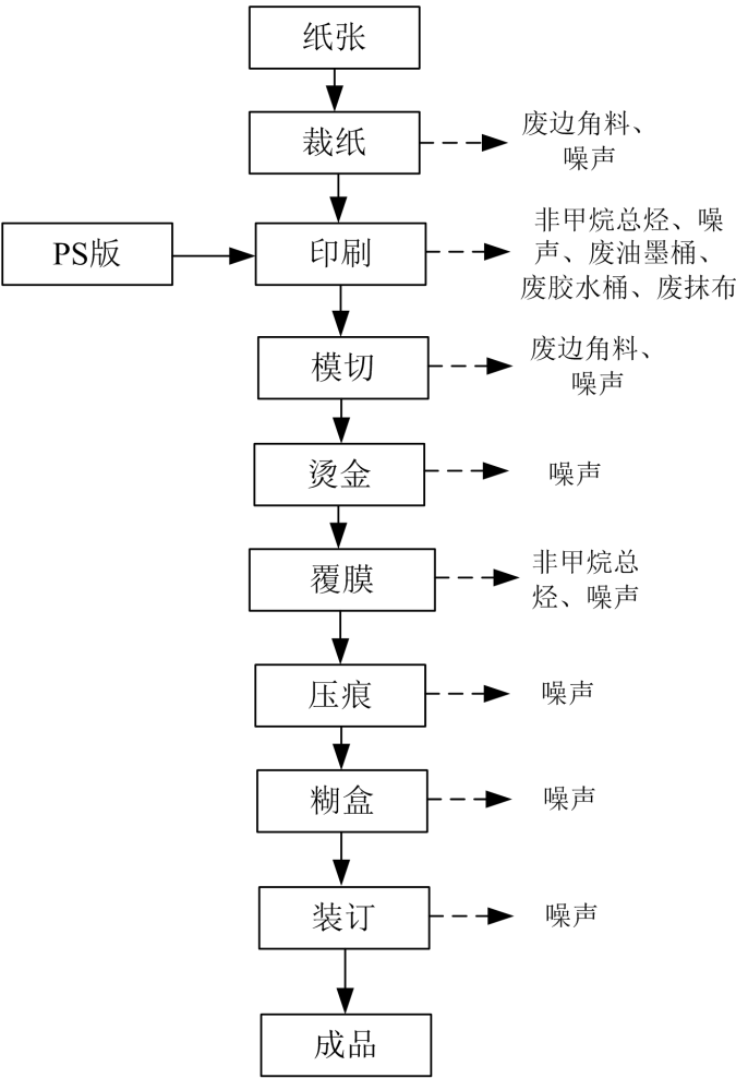
图 1 运营期生产工艺流程及产污环节图
