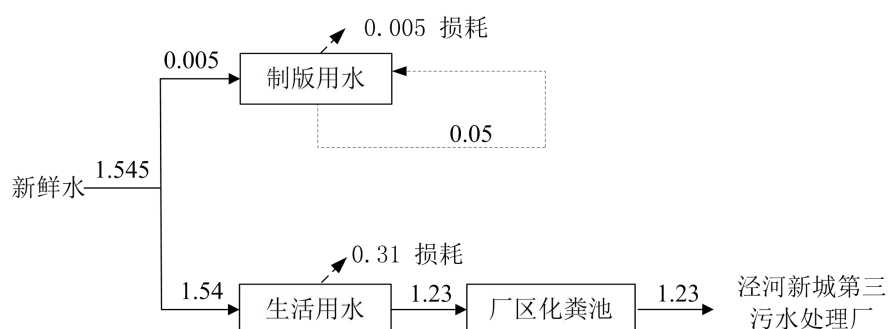
图 2 项目水平衡图 ( \text{m}^3/\text{d} )
