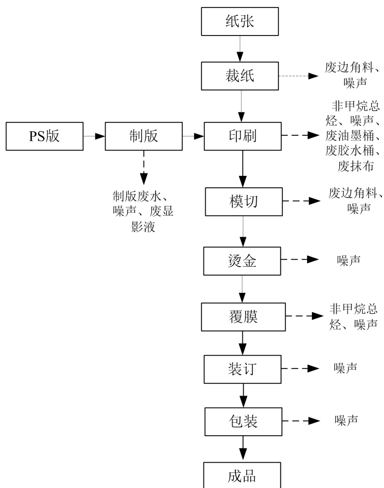
图 1 运营期生产工艺流程及产污环节图
