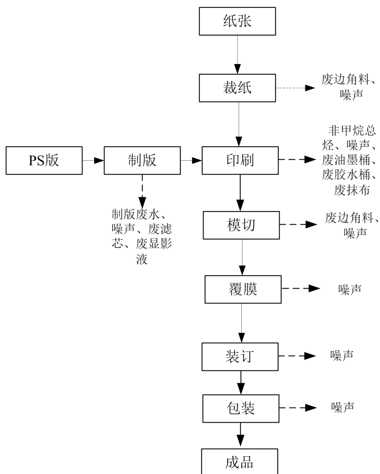
图 1 运营期印刷生产工艺流程及产污环节图
