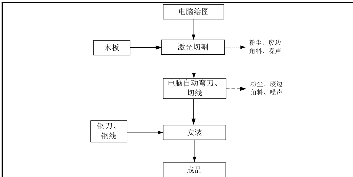
图2 运营期激光刀模生产工艺流程及产污环节图
