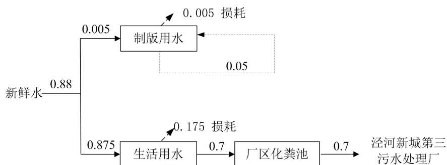
图3 项目水平衡图 (m³/d)
