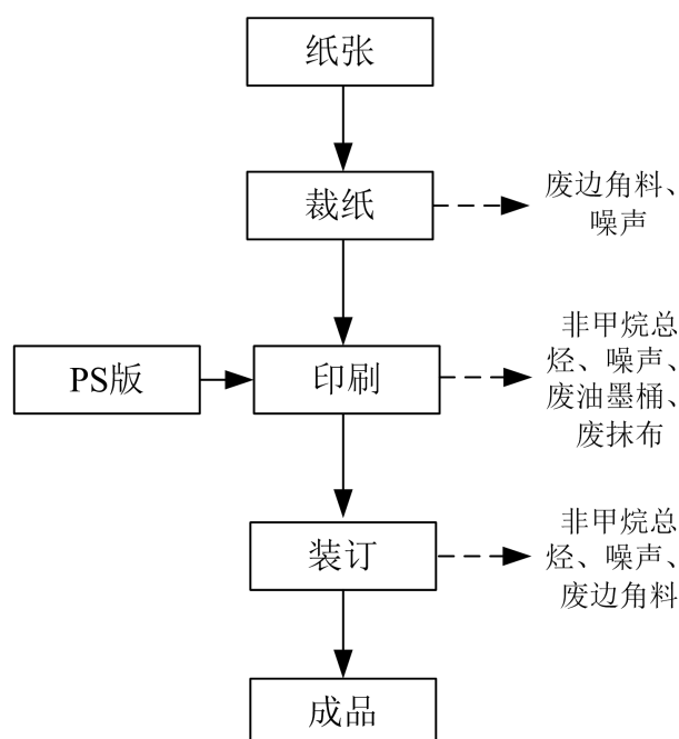
图 1 运营期生产工艺流程及产污环节图
