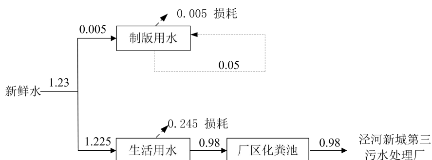
图 2 项目水平衡图 (m 3 /d)
