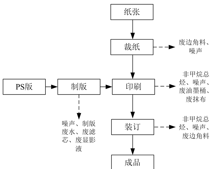
图 1 运营期生产工艺流程及产污环节图
