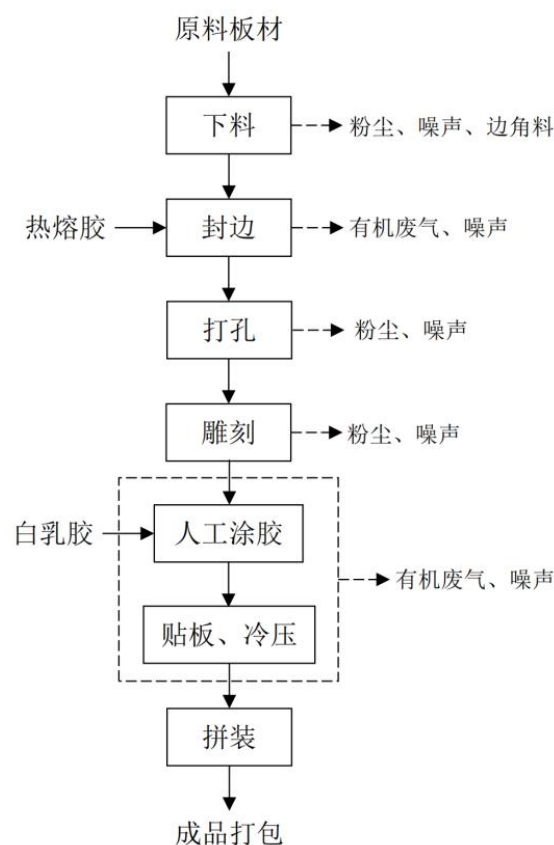
图3 运营期家具工艺流程及产污环节图
