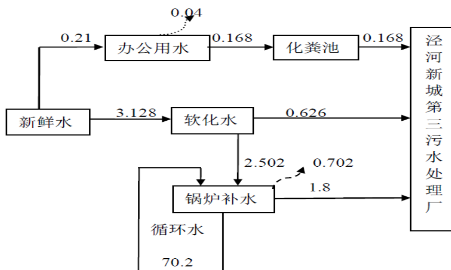
图3 项目水平衡图 单位：m³/d
