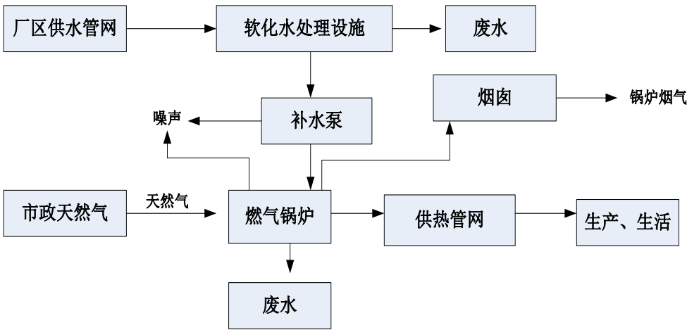
图 1 锅炉燃烧工艺流程及产污环节图
