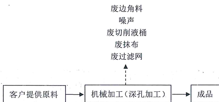
图 2 项目工艺流程及产污环节图
