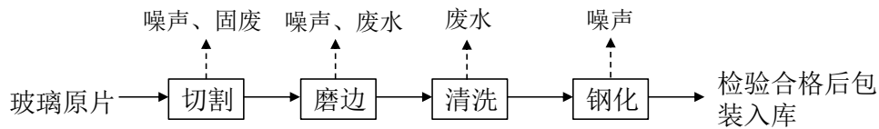
图3 钢化玻璃生产工艺流程及产污节点图
