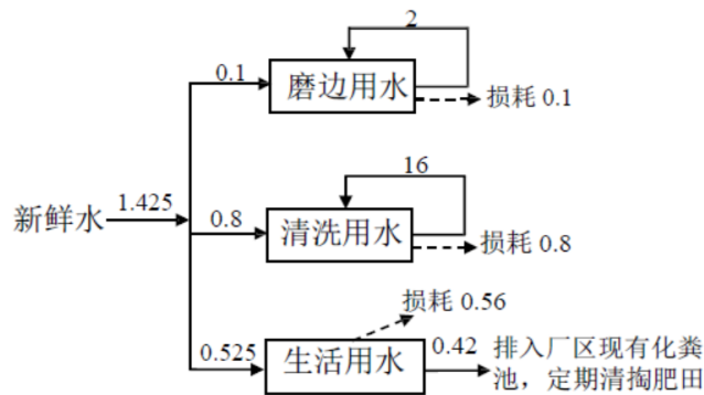
图 1 项目水平衡图（单位： \text{m}^3/\text{d} ）
