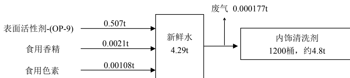
图 1-3 内饰清洗剂物料平衡图 (t/a)
