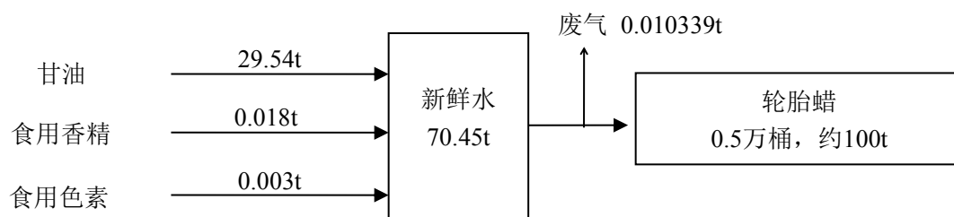
图 1-2 轮胎蜡物料平衡图 (t/a)
