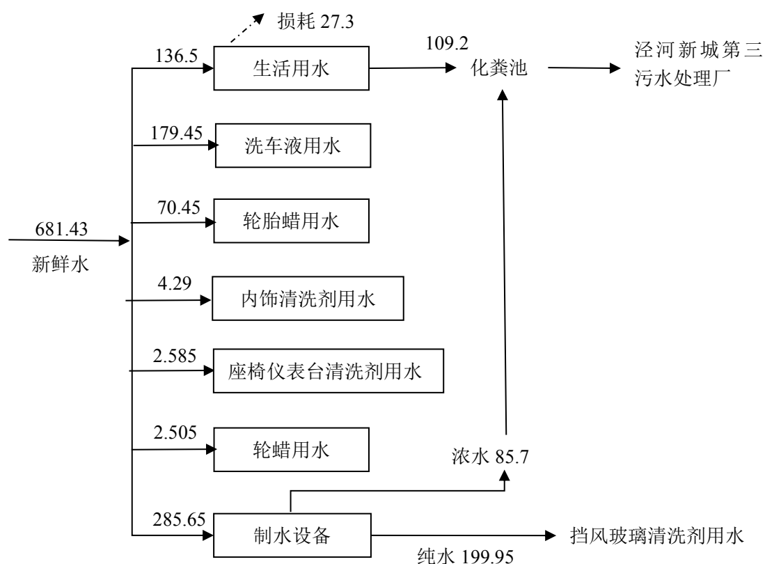
图 1-7 项目水平衡图 单位: t/a
