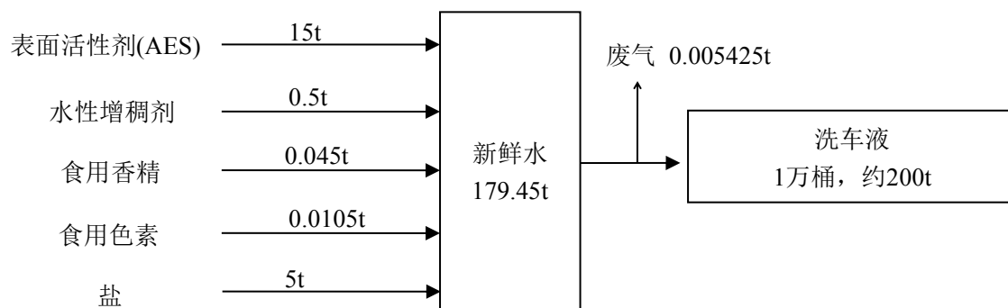
图 1-1 洗车液物料平衡图 (t/a)
