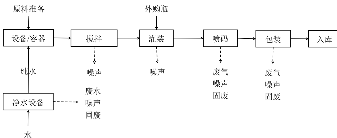
图 5-3 挡风玻璃清洗剂生产工艺及产污环节图
