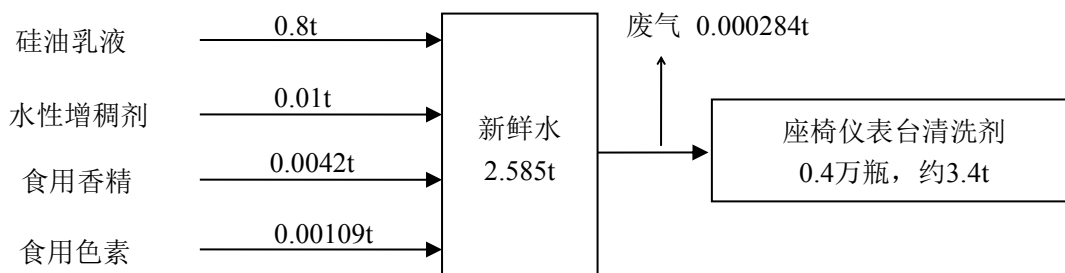
图 1-4 座椅仪表台清洗剂物料平衡图 (t/a)
