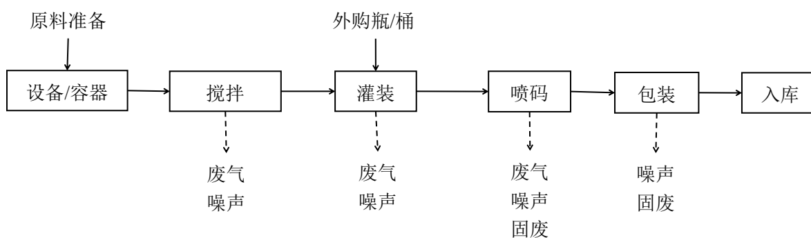
图 5-2 洗车液、轮胎蜡、内饰清洗剂、座椅仪表台清洗剂、车蜡生产工艺及产污环节图
