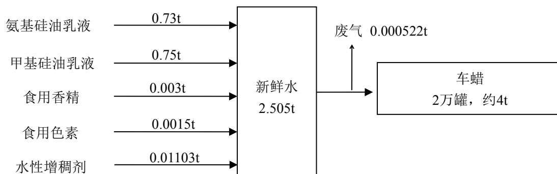
图 1-5 车蜡物料平衡图 (t/a)
