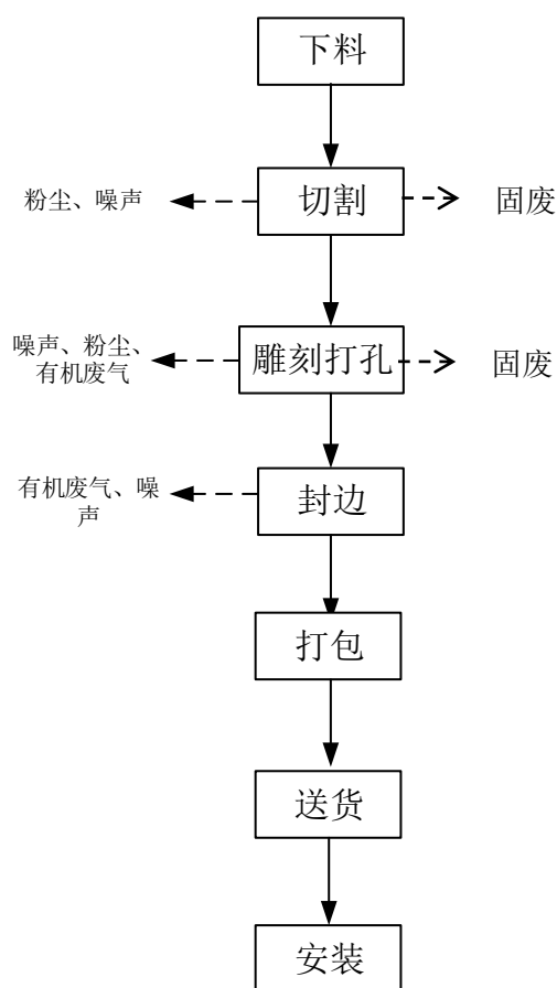
图 3 生产工艺流程及主要产排污节点图
