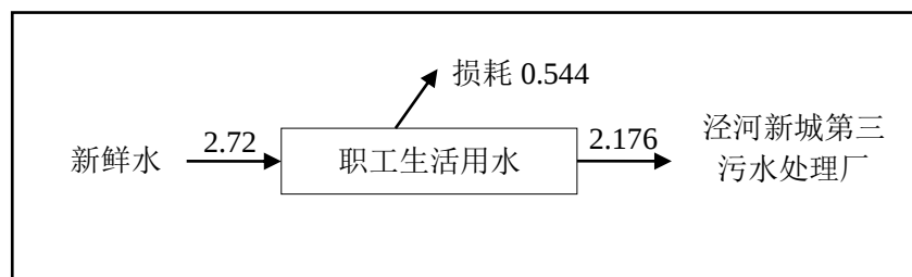
图 2 建设项目水平衡图 单位：m 3 /d
