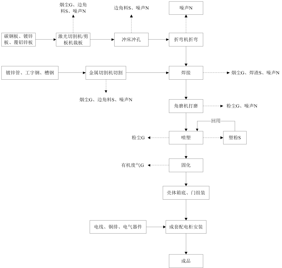
图5-2 运营期生产工艺流程及产污节点图
