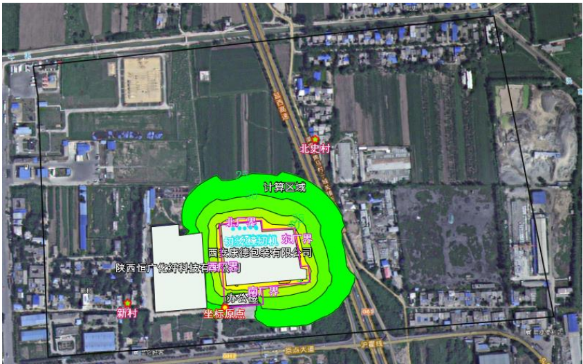
图 5 昼间噪声贡献等值线图
