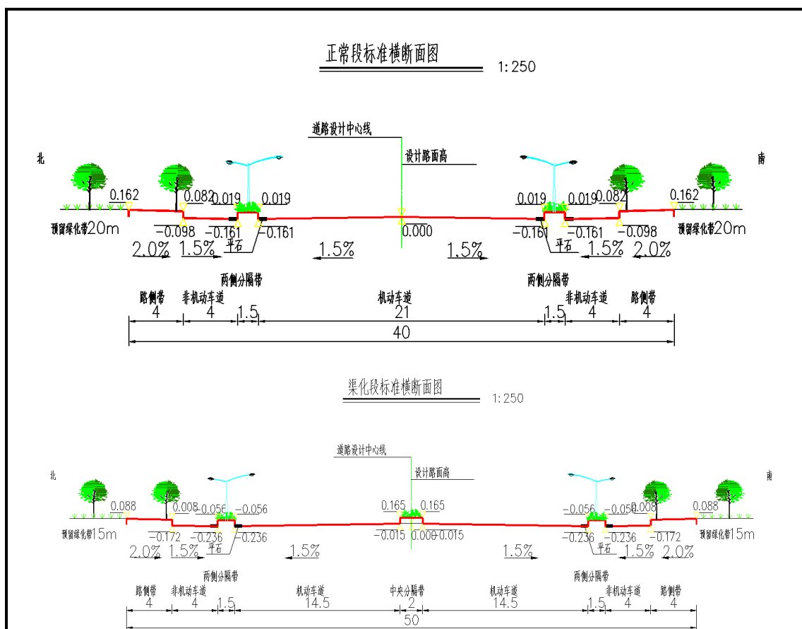
图1 项目标准横断面结构图
