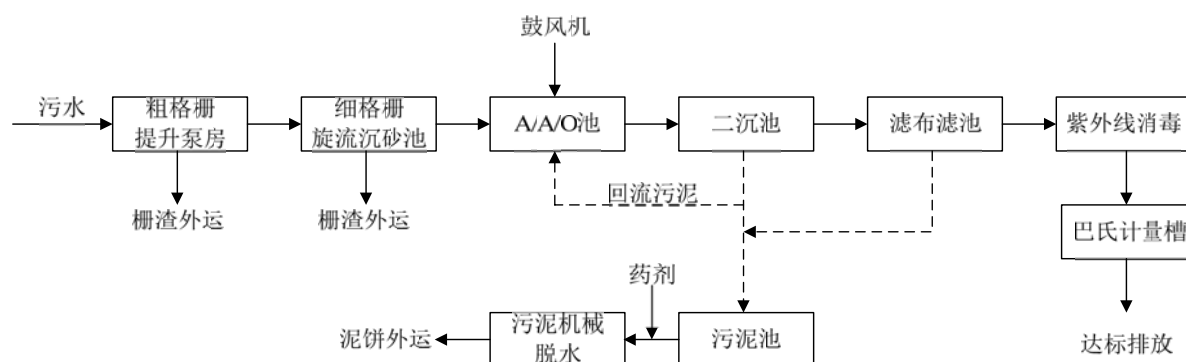
图 3 泾河第二污水处理厂污水处理工艺流程图
