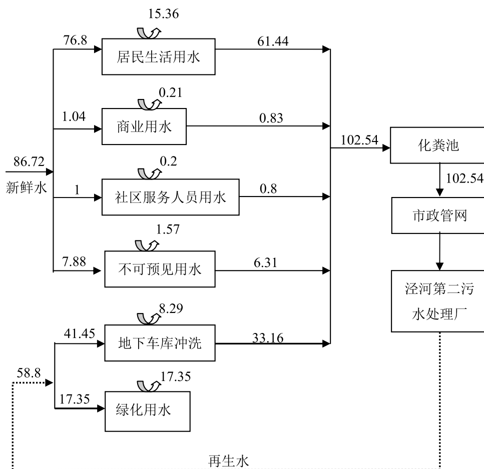
图2 本项目水平衡及污水走向图 单位: \text{m}^3/\text{d}
