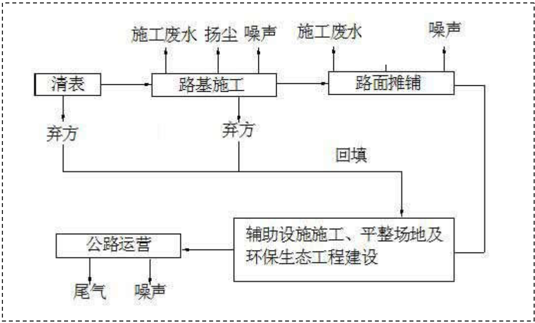
图 4 道路建设、运输流程及产污节点图
