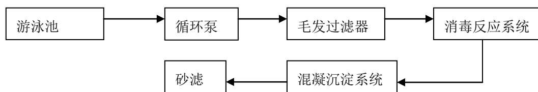
图 1 循环水处理工艺
