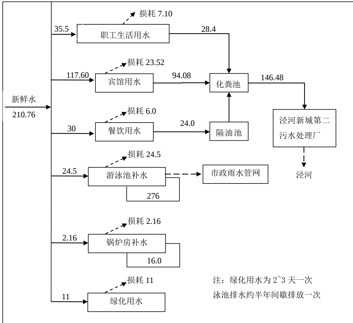
图 2 本项目水平衡图 单位 m 3 /d
