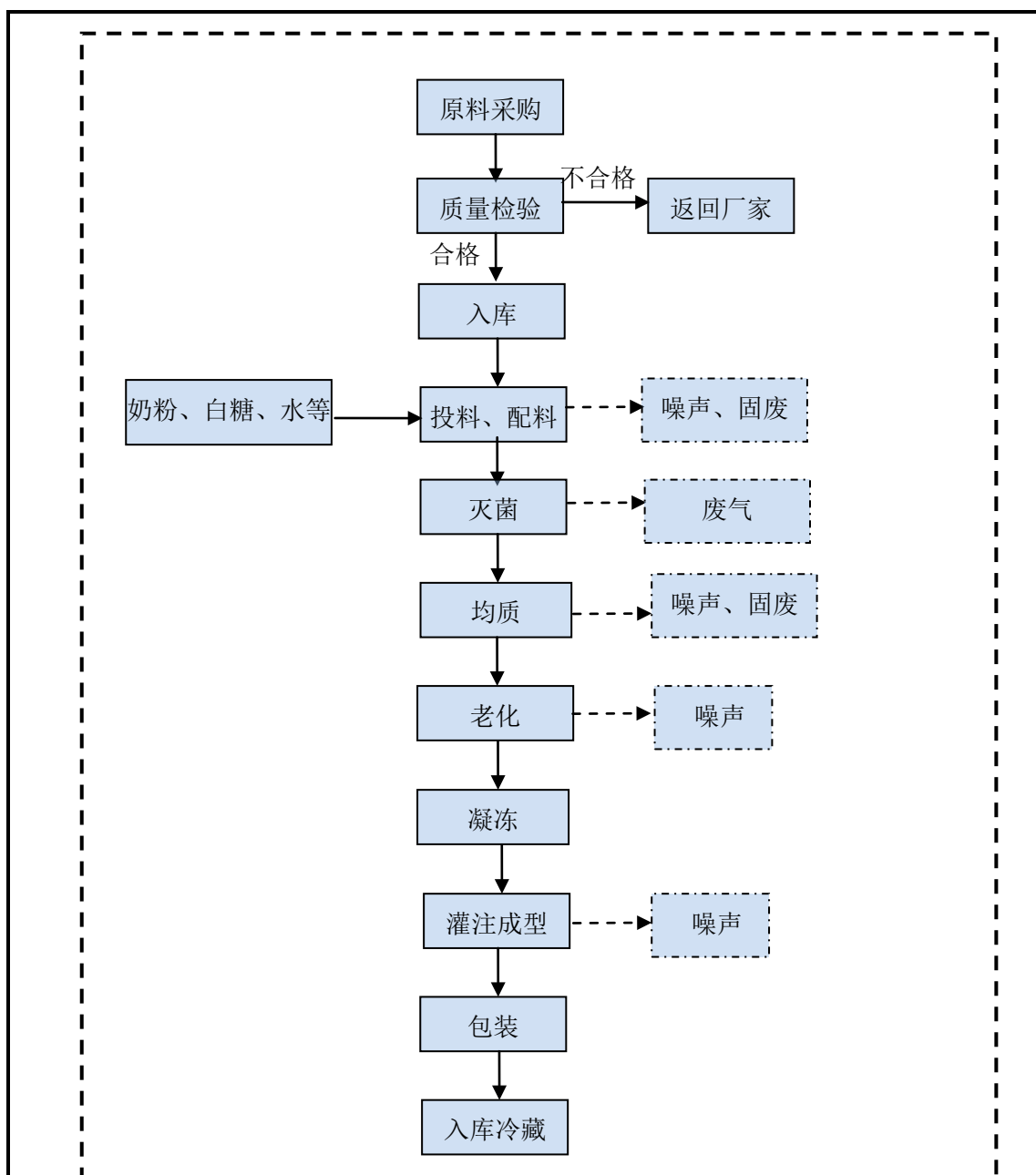
图 3 项目工艺流程及产污环节分析图
