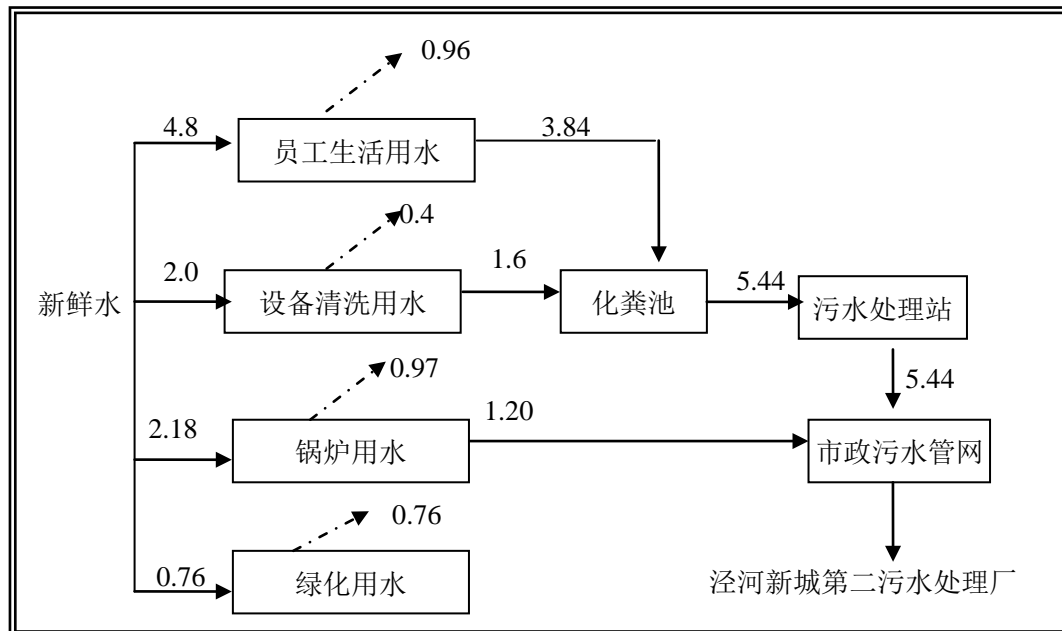
图 4 项目用水平衡图 (m 3 /d)
