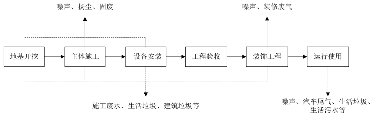
图 1 工艺流程及产污情况图
