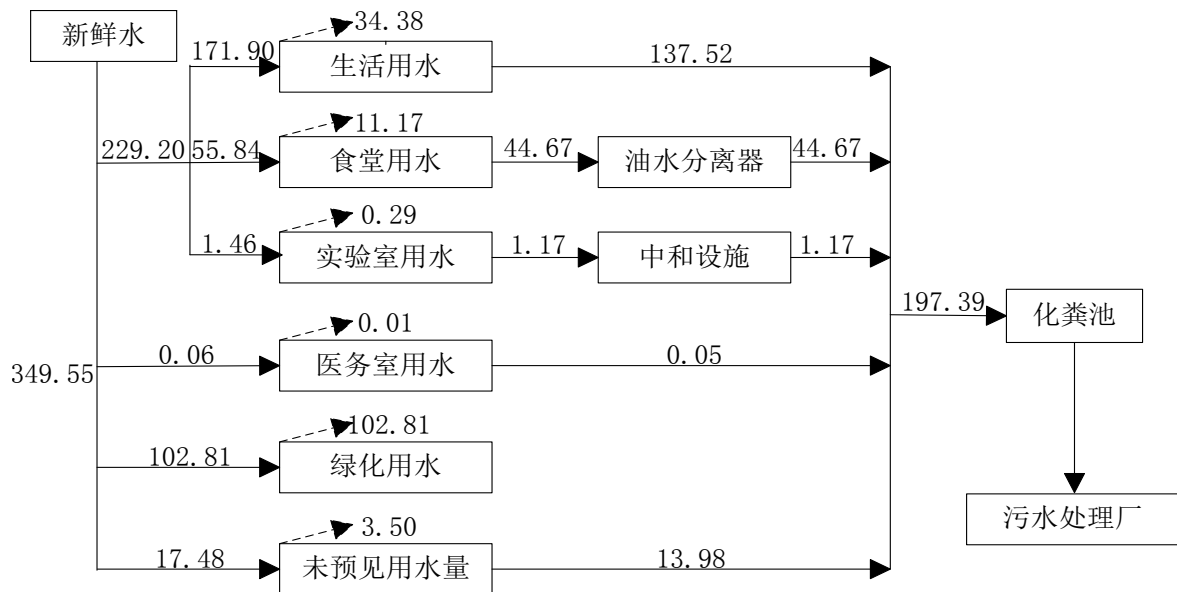
图 2 水平衡图 单位：m 3 /d
