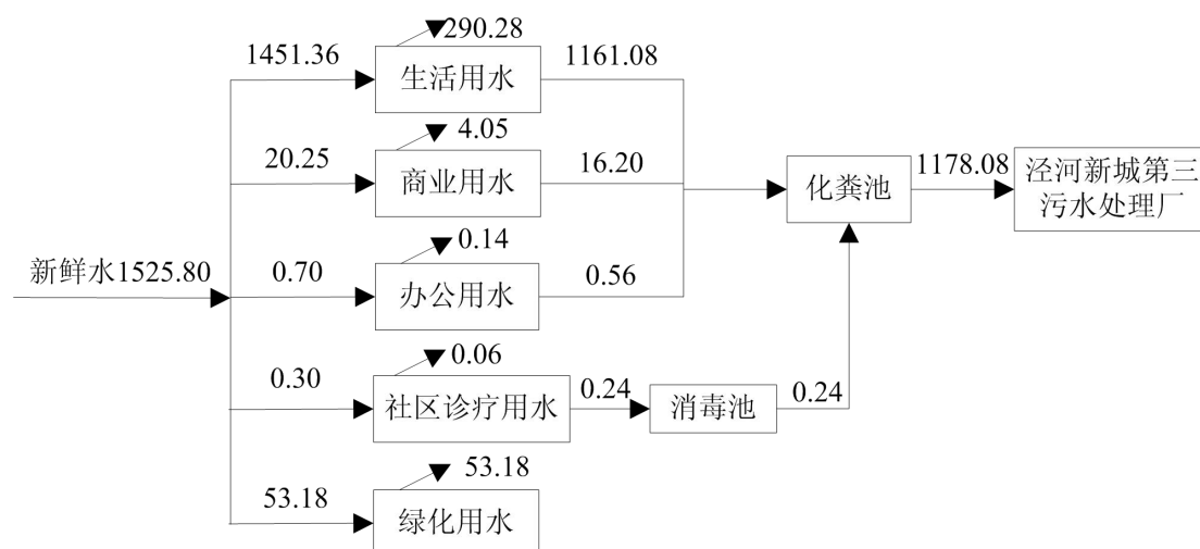
图 2 水平衡图
