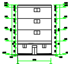
站房侧立面图 1:100
