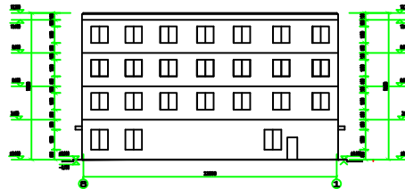
站房背立面图 1:100
