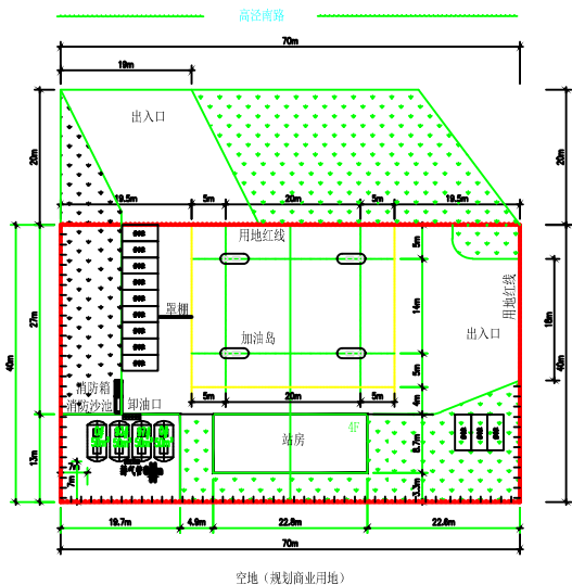
泾阳县崇宋加油站总平面图
