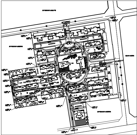
原总平面图
