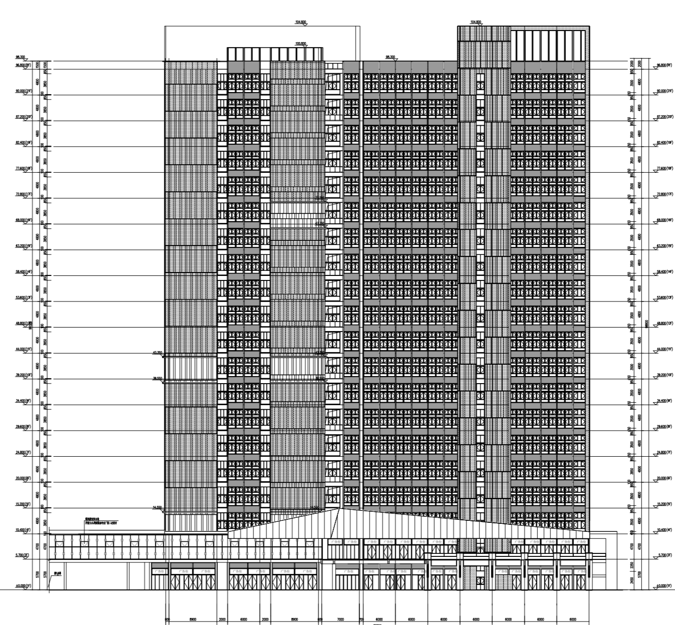
3#楼西立面
