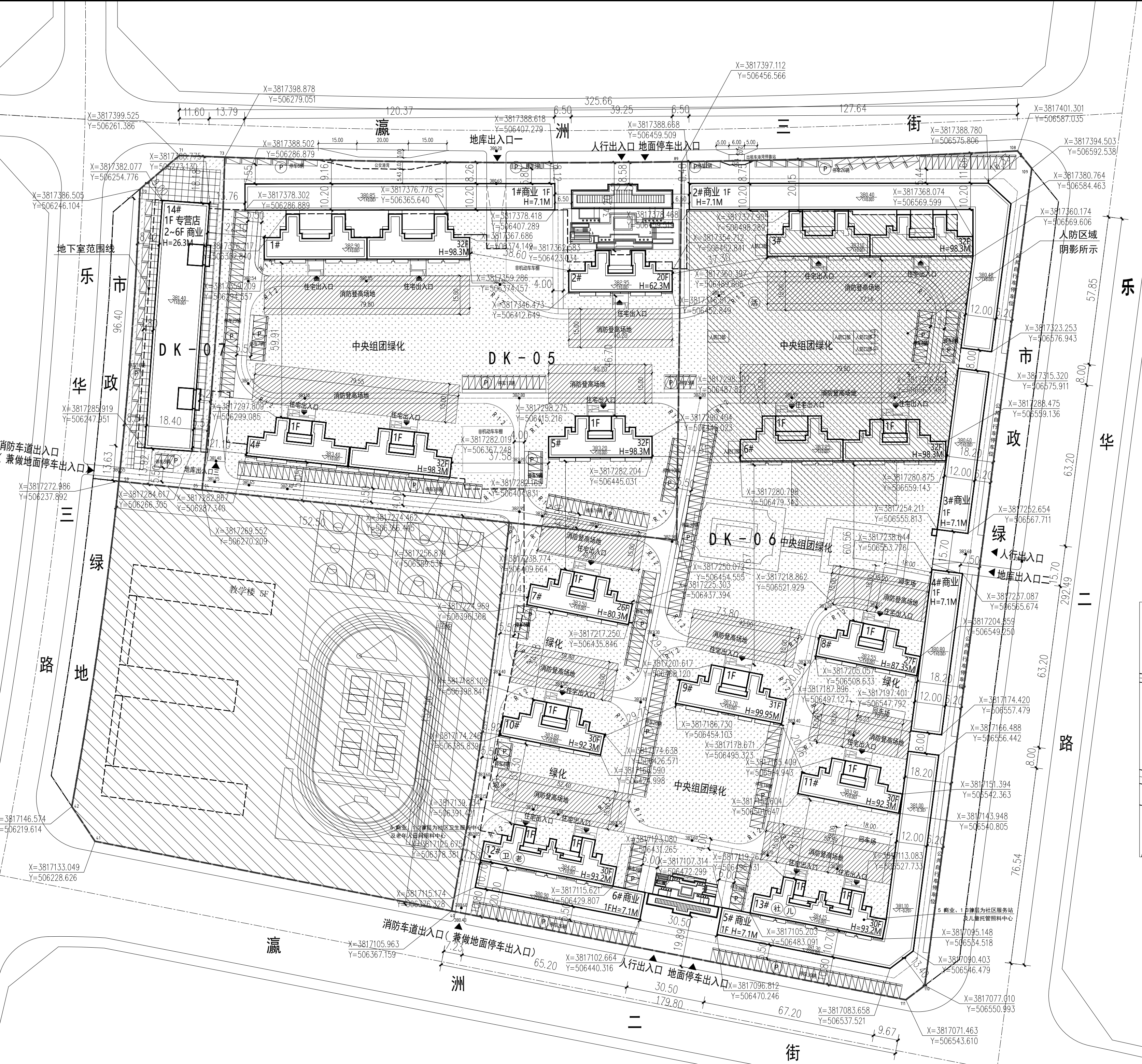
总平面图 1 : 1 0 0 0
